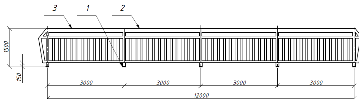
Рисунок 1. – Внешний вид перильного ограждения из стеклопластика на трассе обход г. Брянска, путепровод на 21 км, производство АО «Флотенк», и поэлементная монтажная схема (1 – траверса-крепление к плите проезжей части, 2 – центральные монолитные перила из стеклопластика, 3 – крайние монолитные перила из стеклопластика). (Составлен авторами)
