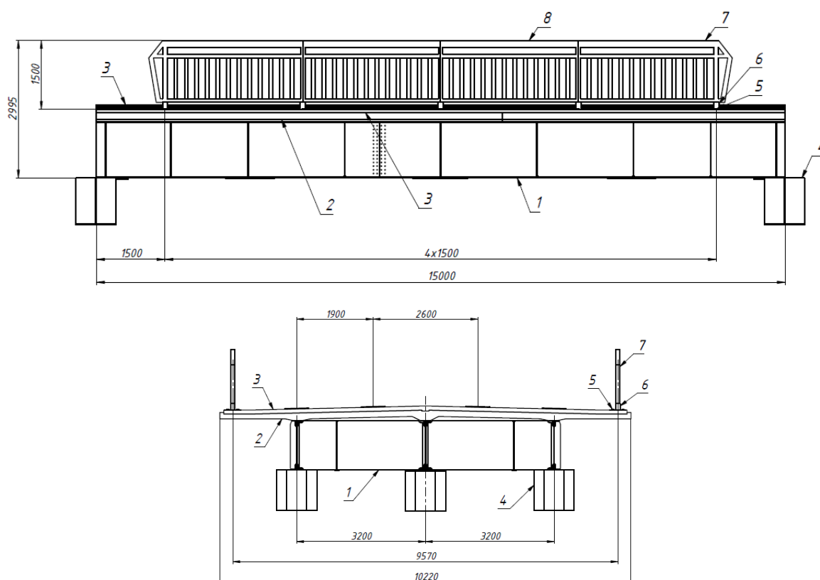
Рисунок 5. Внешний вид и поэлементный чертеж серийного мостового сооружения со стеклопластиковым перильным ограждением (1 – пролетное строение, 2 – ж/б плита проезжей части, 3 – асфальтобетонное покрытие, 4 – опорный ж/б столб, 5 – анкерный болт, 6 – траверса анкерного крепления, 7 – крайний элемент стеклопластикового ограждения, 8 – средний элемент стеклопластикового ограждения). Составлен авторами.
